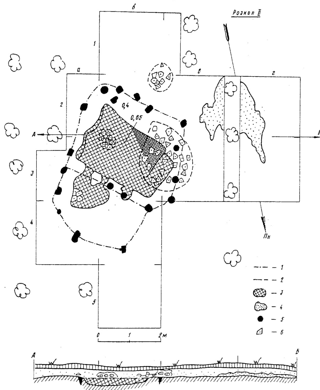
Locuință de suprafață de la Gorodnitsa (după Крушельницкая 1993)
