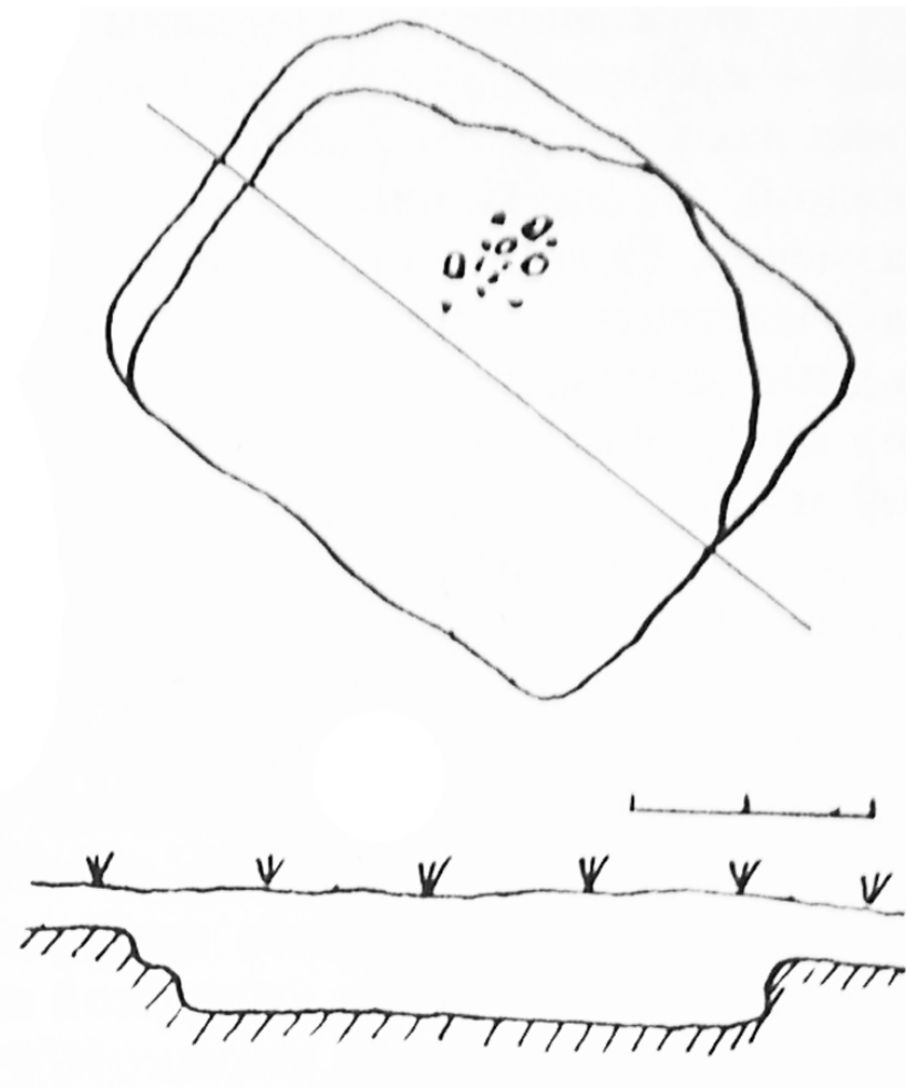
Locuințe adâncite de la Krivče și Lisičniki (după Крушельницкая, Малеев 1990)
