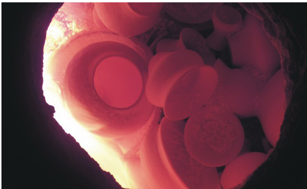
Imagine din timpul arderii experimentale a ceramicii (Experimentul Cucuteni, România)
